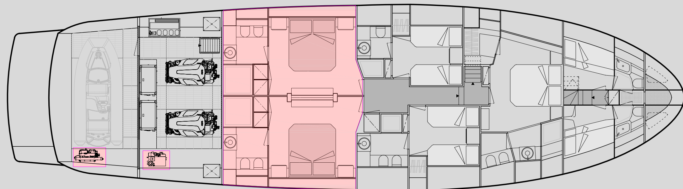
НИЖНЯЯ ПАЛУБА
